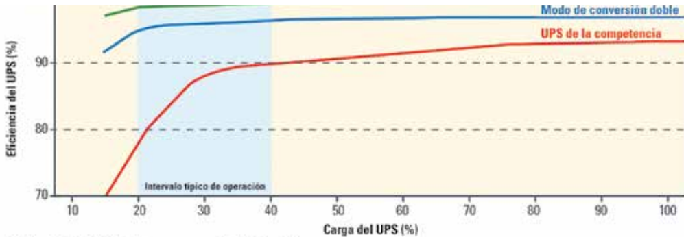
Eficiencia del 93PM de Eaton en conversión doble y ESS
